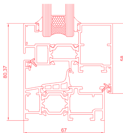
Sección vertical
