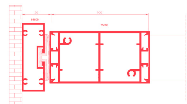
Secciones horizontales
