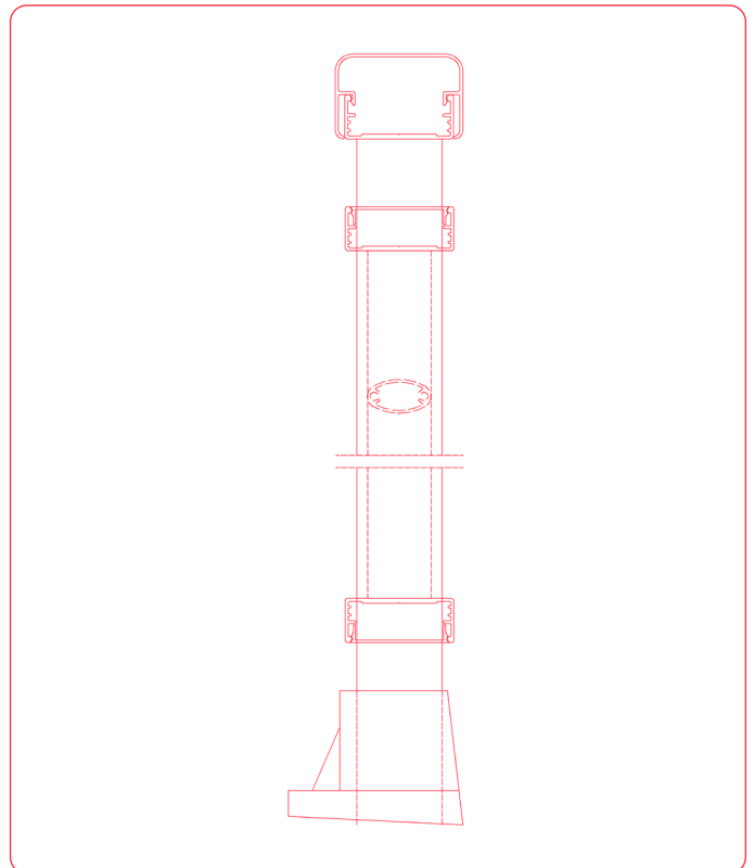
Barrotes con doble pasamanos
