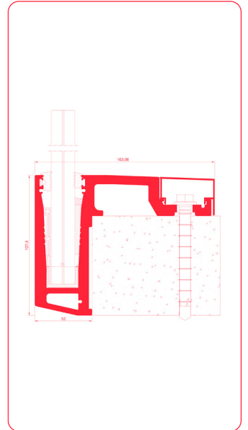
Montaje a canto forjado
