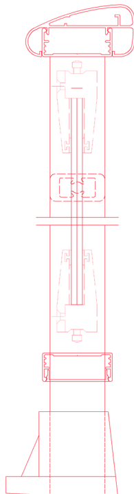
Vidrio con pinza vertical
