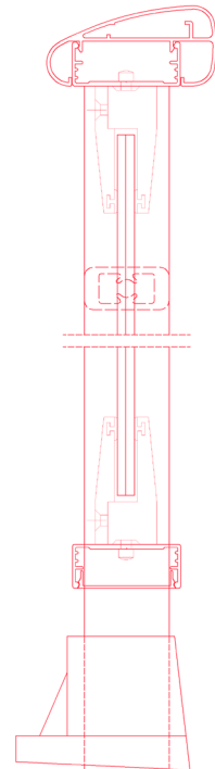
Vidrio con pinza horizontal
