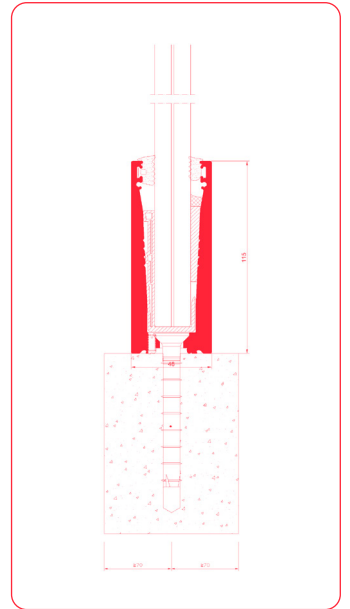
Montaje sobre forjado
